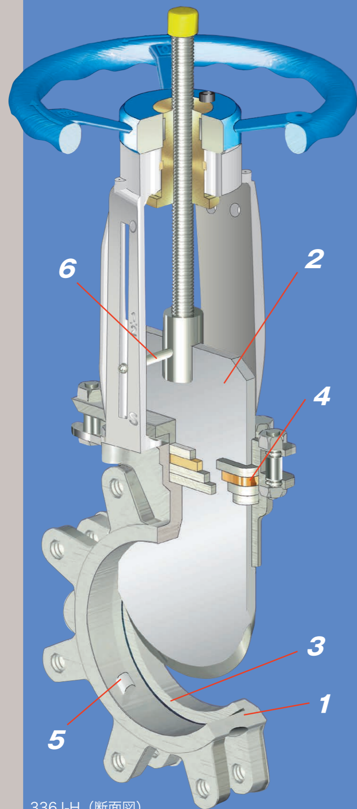
336J-H (断面図)
